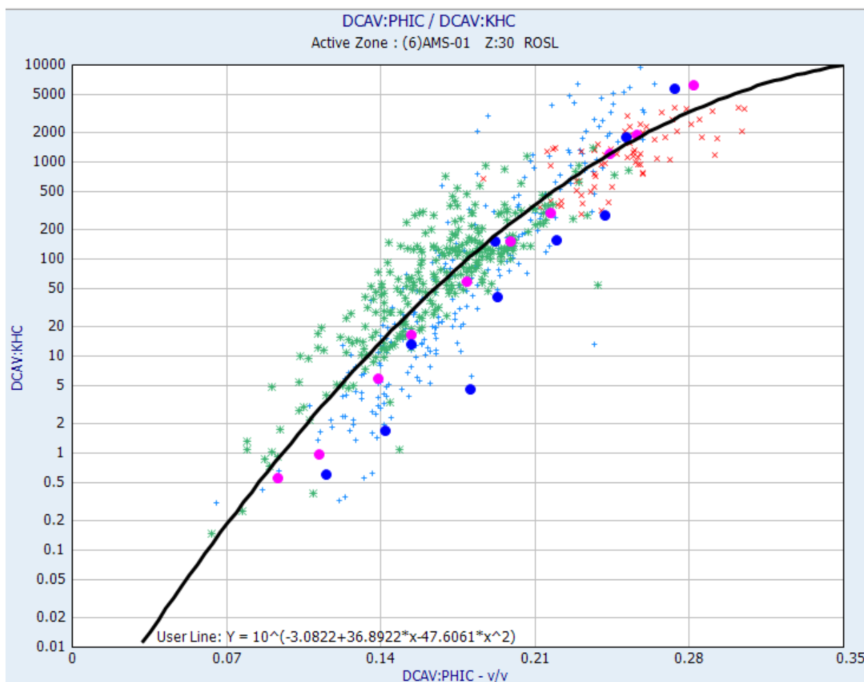
Figuur 3-7: Overburden gecorrigeerde kern gas permeabiliteit (KHC) tegenover overburden gecorrigeerde boorkernporositeit (PHIC) in ROSL voor drie SCAN-putten: AMS-01 (blauw kruis), BLT-01 (groen kruis) & EDE-01 (rode x). Daarnaast worden de gemeten permeabiliteit voor gas onder spanning (magenta stip) en voor brijn onder spanning (blauwe stip) weergegeven ten opzichte van de porositeit onder spanning van put AMS-01. Over de gegevens heen (zwarte lijn) is de poro-perm regressiefunctie (alle boorkernputten) weergegeven die voor de ROSL is afgeleid.
