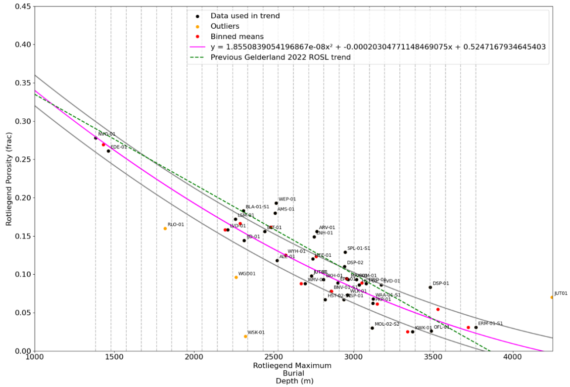
Figuur 4-5: Porositeit-diepte trend voor de Formatie van Slochteren reservoir (Rotliegend), met behulp van de lokale uniforme begravingslijn die in dit onderzoek is gegenereerd (zie het hoofdstuk 3.4 over petrofysica voor meer informatie).
