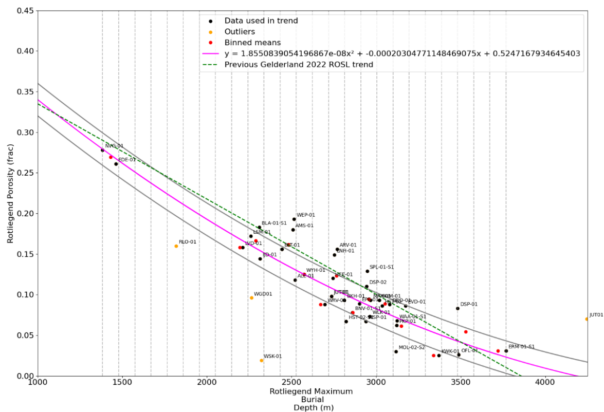
Figuur 3-16: Grafiek die de porositeit-diepte trend voor de Formatie Slochteren (ROSL) (Rotliegend Groep) weergeeft, gebruikmakend van de voor opheffing gecorrigeerde gemiddelde reservoirdieptes.
