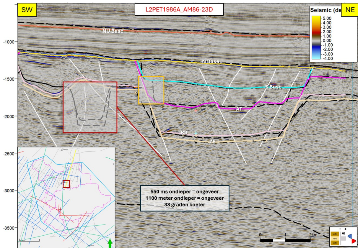
Figuur 2-10: Seismische lijn L2PET1986A_AM86-23D illustreert de vergelijking tussen legacy (zwarte stippellijn) en bijgewerkte (gekleurde) interpretaties. Er zijn opvallende lokale verbeteringen waarneembaar rond breuken, met verschillen van wel 550 ms. De sectie toont ook een afsnijding van de Basis Schieland (S) en Basis Altena (AT) horizonten door de Basis N-discordantie.
