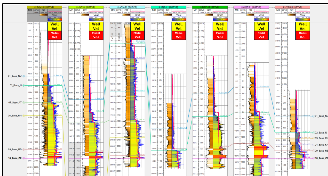
Figuur 2-16: Vergelijking van de werkelijke acoustic putsnelheid berekend op basis van sonic logs (linker groenblauwe curve) en TNO-modelsnelheden (rode lijn). Putlogs zijn genivelleerd langs het Top Formatie van Slochteren (= Basis Zechstein Groep).
