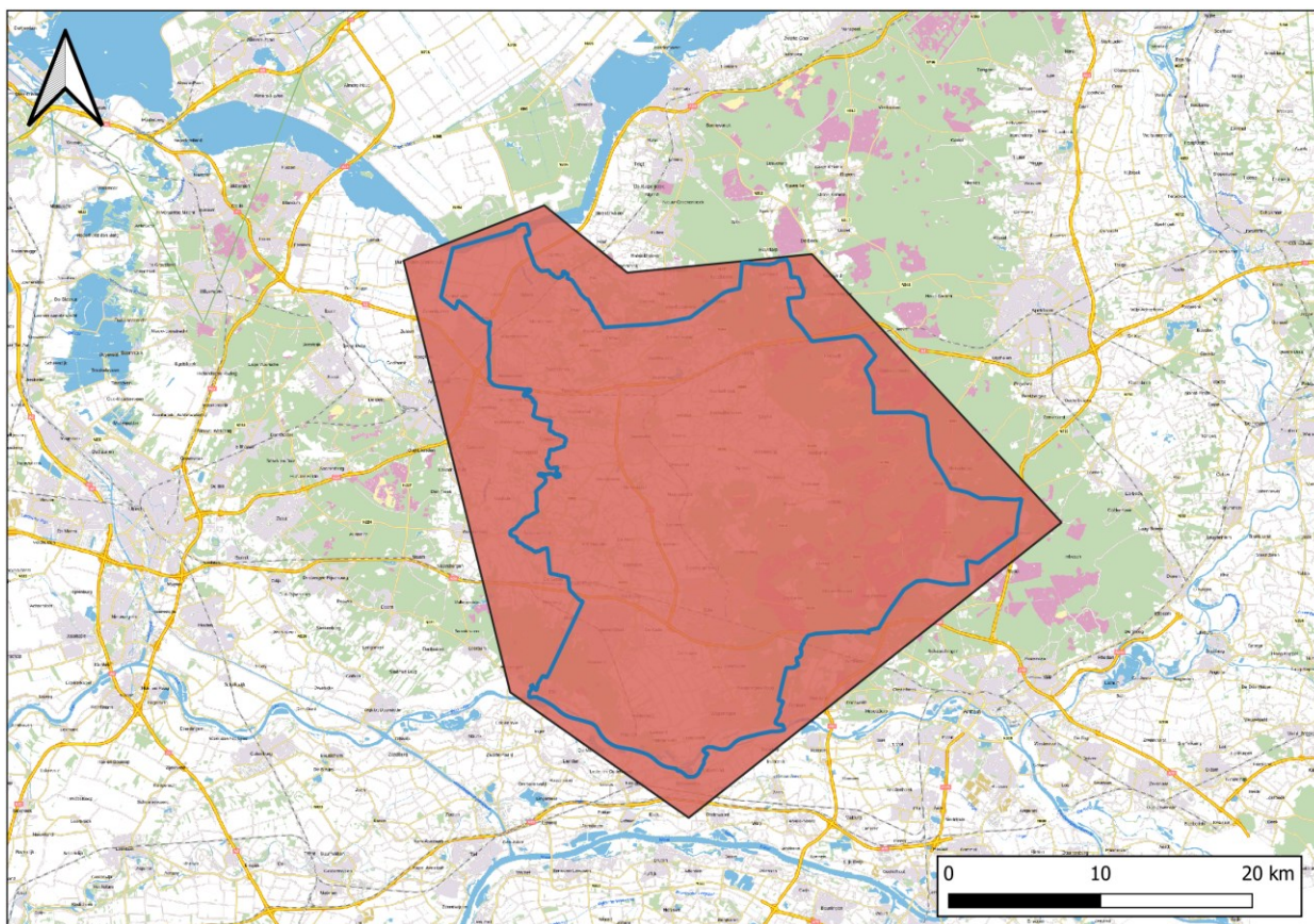
Figuur 6-3: Kaart van het risico op aanwezigheid van voldoende dikke Onder Volpriehausen-reservoirs. Rood = hoog risico (<40 m dikte), geel = matig risico (40–70 m), groen = niet aanwezig. Blauwe lijn = provinciale grens.
