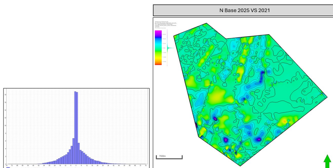
Figuur 2-5. Basis Noordzee Supergroep (N). Vergelijking tussen de seismische interpretatie van 2025 en het oude raster. Warme kleuren geven gebieden aan waar de bijgewerkte interpretatie dieper is, terwijl koude kleuren gebieden aangeven waar deze ondieper is. Het histogram aan de linkerkant illustreert de verdeling van diepteverschillen (ms) over het onderzoeksgebied.
