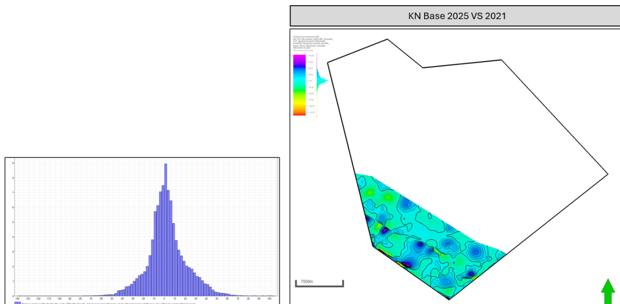
Figuur 2-7: Basis Rijnland (KN). Vergelijking tussen de seismische interpretatie voor 2025 en het oude raster. Warme kleuren geven gebieden aan waar de bijgewerkte interpretatie dieper is, terwijl koude kleuren gebieden aangeven waar deze ondieper is. Het histogram aan de linkerkant illustreert de verdeling van diepteverschillen (ms) over het onderzoeksgebied.
