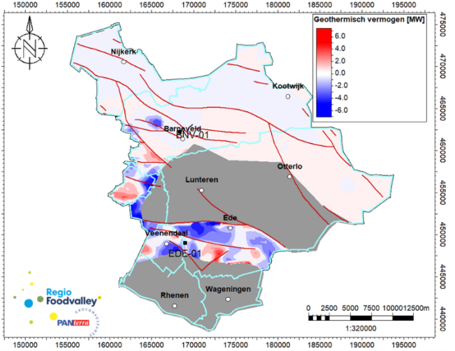
Vergelijking vermogenskaart bij 35 °C injectie (ROSL - Middel scenario)
