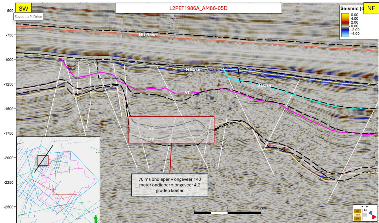
Figuur 2-9: Seismische lijn L2PET1986A_AM86-05D illustreert de vergelijking tussen legacy (zwarte stippellijn) en bijgewerkte (gekleurde) interpretaties. Er zijn opvallende lokale verbeteringen waarneembaar rond breuken, met 50-100 ms verschil. De sectie toont ook de afsnijding van de Base Schieland (S) en Base Altena (AT) horizonten door Basis N-discordantie.
