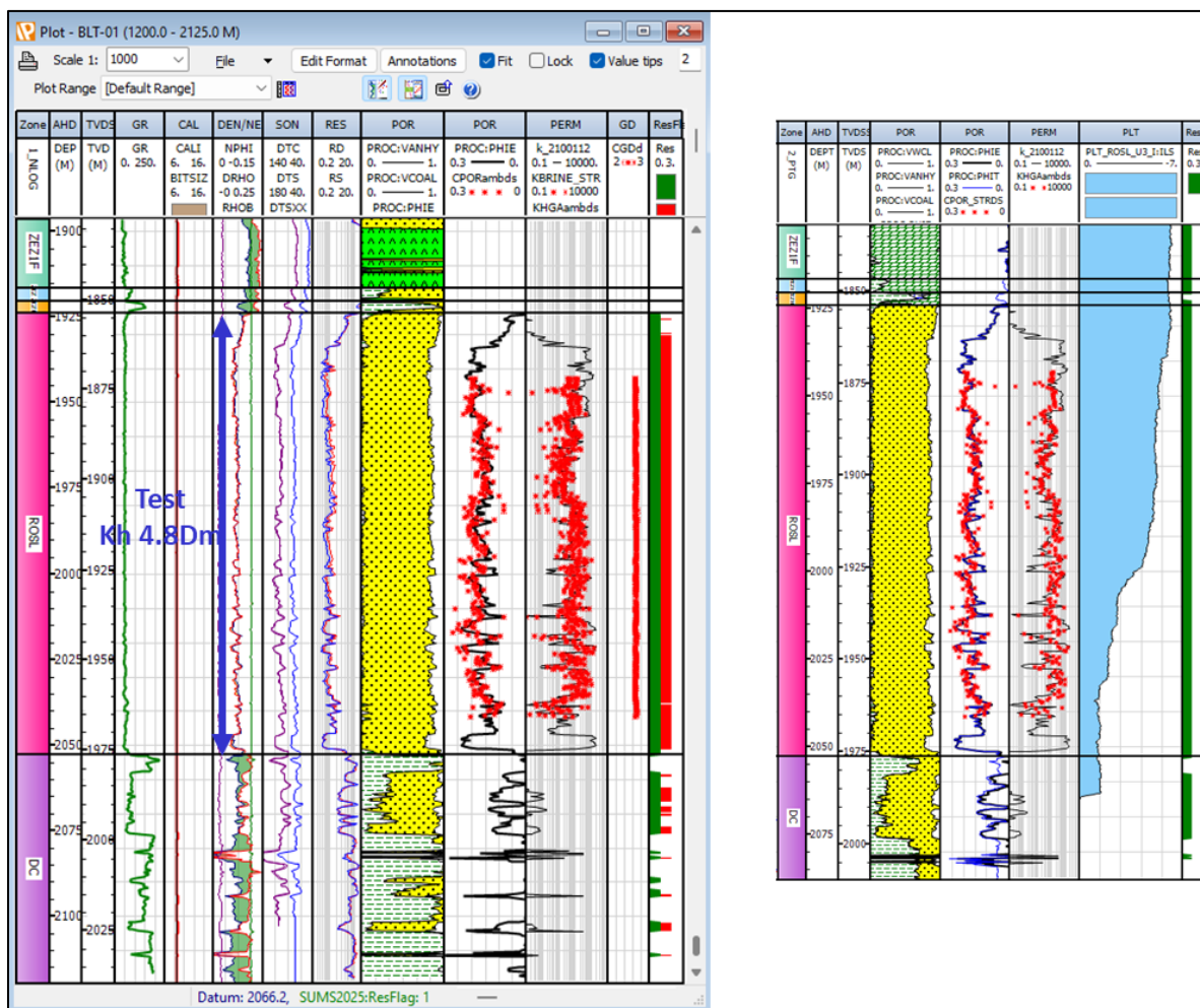
Figuur 3-23: Logplot van ROSL-interval in BLT-01 waarbij het geteste interval (118 m) en geïnterpreteerde Kh links worden weergegeven, en rechterkant weergeeft PLT-injectieprofiel tijdens de test.
