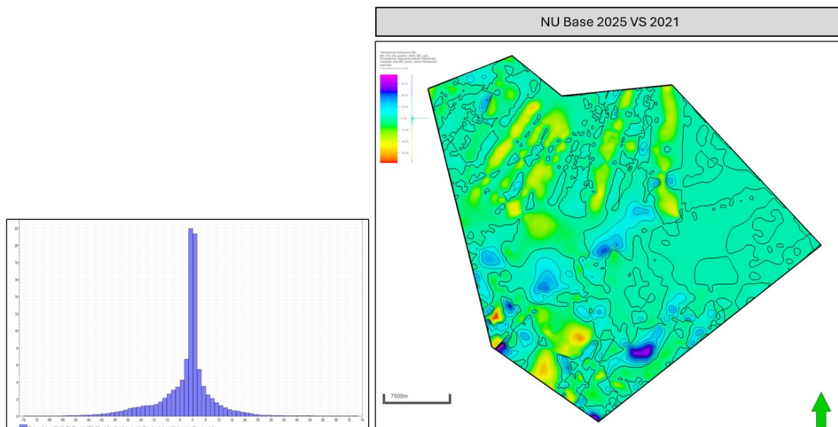
Figuur 2-4: Basis Boven-Noordzee Groep (NU). Vergelijking tussen de seismische interpretatie van 2025 en het oude raster. Warme kleuren geven gebieden aan waar de bijgewerkte interpretatie dieper is, terwijl koude kleuren gebieden aangeven waar deze ondieper is. Het histogram aan de linkerkant illustreert de verdeling van diepteverschillen (ms) over het onderzoeksgebied.
