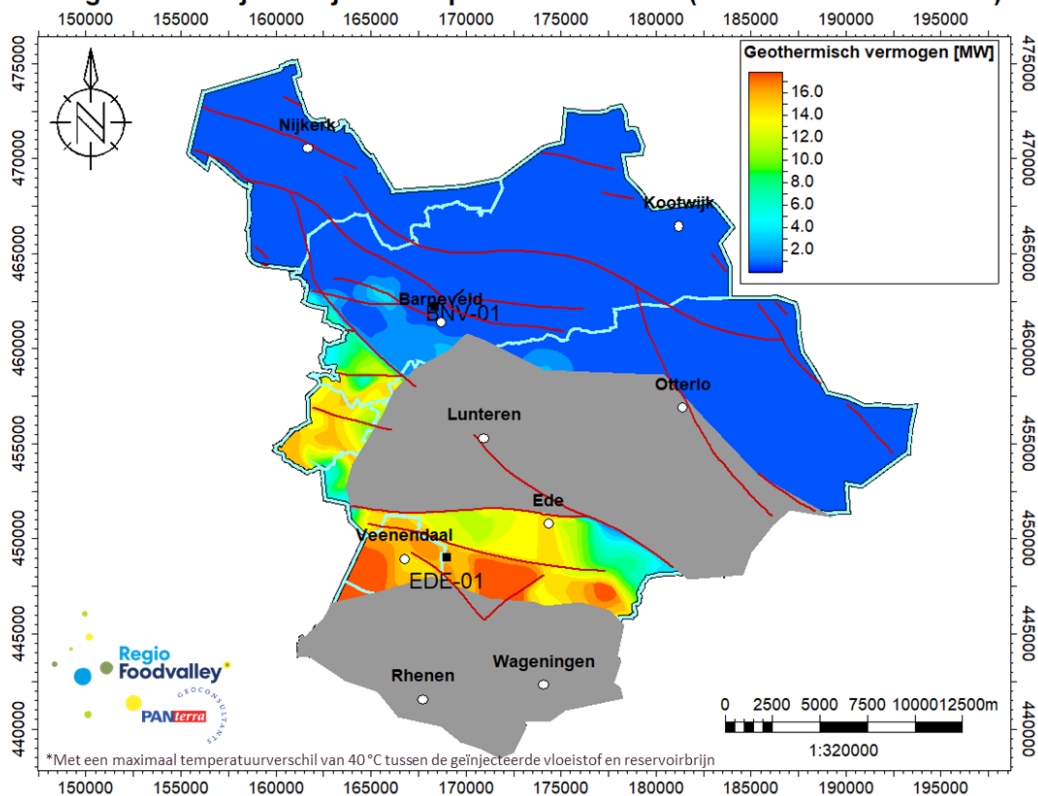
Figuur 5-5: Vermogenskaart voor de Formatie van Slochteren reservoir in het middelsenario. Rode lijnen geven breuken weer; grijze vlakken markeren gebieden waar de Formatie van Slochteren reservoir ontbreekt (op basis van seismische lijnen).
