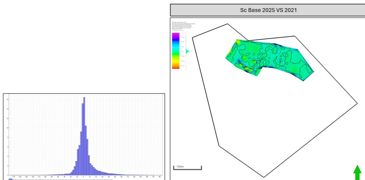
Figuur 2-8: Basis Schieland. Vergelijking tussen de seismische interpretatie van 2025 en het oude raster. Warme kleuren geven gebieden aan waar de bijgewerkte interpretatie dieper is, terwijl koude kleuren gebieden aangeven waar deze ondieper is. Het histogram aan de linkerkant illustreert de verdeling van diepteverschillen (ms) over het onderzoeksgebied.
