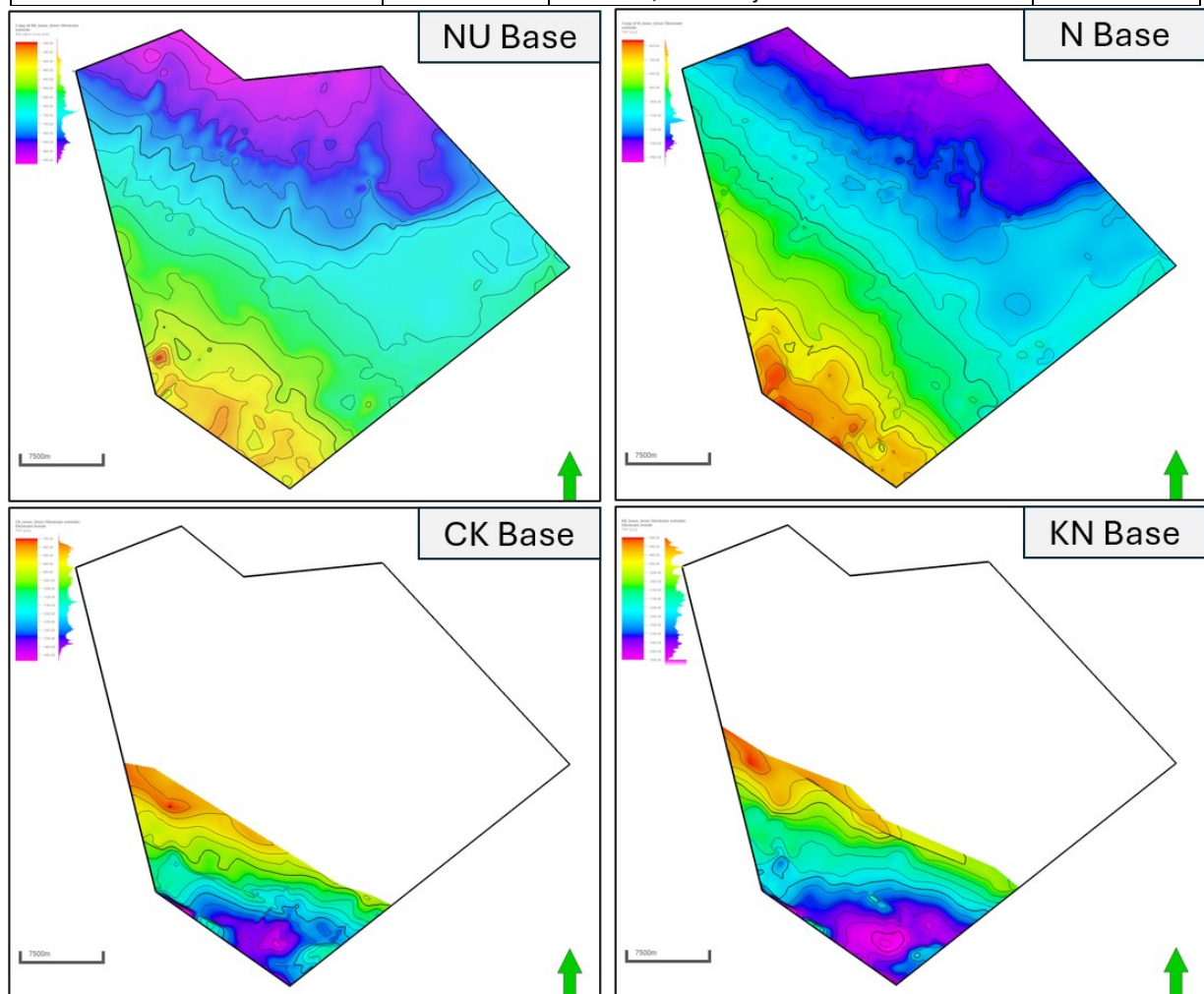
Figuur 2-2: Resultierende grids in het tijdsdomein (ms) voor Basis Boven-Noordzee Groep (NU), Basis Noordzee Groep (N), Basis Krijt-kalk Groep (CK) en Basis Rijnland Groep (KN).
