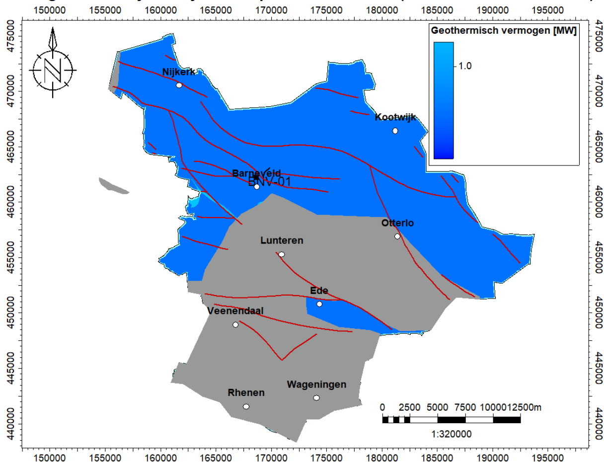
Figuur 5-3. Vermogenskaart in het middel scenario het Onder Volpriehausen Laagpakket. Er wordt een minimale injectietemperatuur van 15 °C gebruikt en een maximaal temperatuurverschil van 40 °C tussen de geïnjecteerde en geproduceerde brijn.
