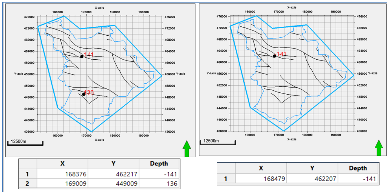
Figuur 2-19: Basiskaart van putten met berekend diepteverschil tussen welltops van het Top Rotliegend (links) of Top Trias (rechts) en de overeenkomstige dieptehorizonten na diepteconversie. De dikke blauwe veelhoek geeft het gebied aan van de snelheidsmodellering in het Foodvalley-projectgebied; de dunne blauwe lijn geeft de grens van Regio Foodvalley aan; en de zwarte lijnen geven breuklocaties aan.
