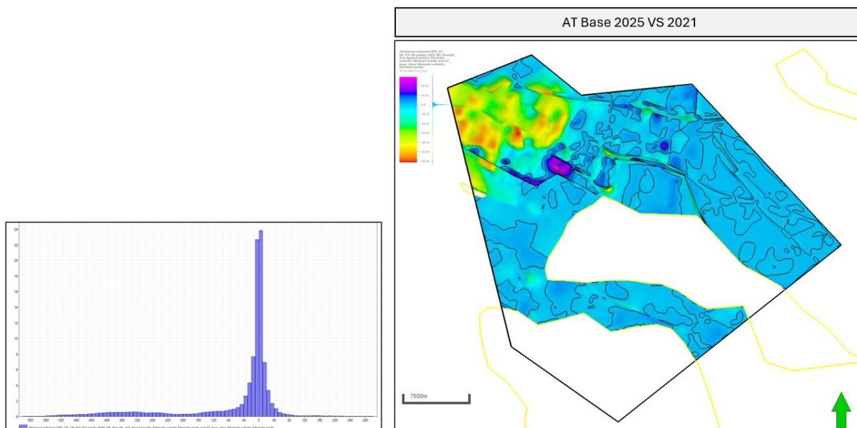
Figuur 2-11: Basis Altena Groep (AT). Vergelijking tussen de seismische interpretatie van 2025 en het oude raster. Warme kleuren geven gebieden aan waar de bijgewerkte interpretatie dieper is, terwijl koude kleuren gebieden aangeven waar deze ondieper is. Het histogram aan de linkerkant illustreert de verdeling van diepteverschillen (ms) over het onderzoeksgebied.
