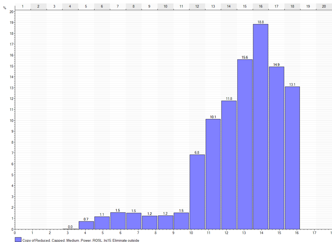
Figuur 5-13: Verdeling van geothermische vermogens dat mogelijk is in prospect 5.
