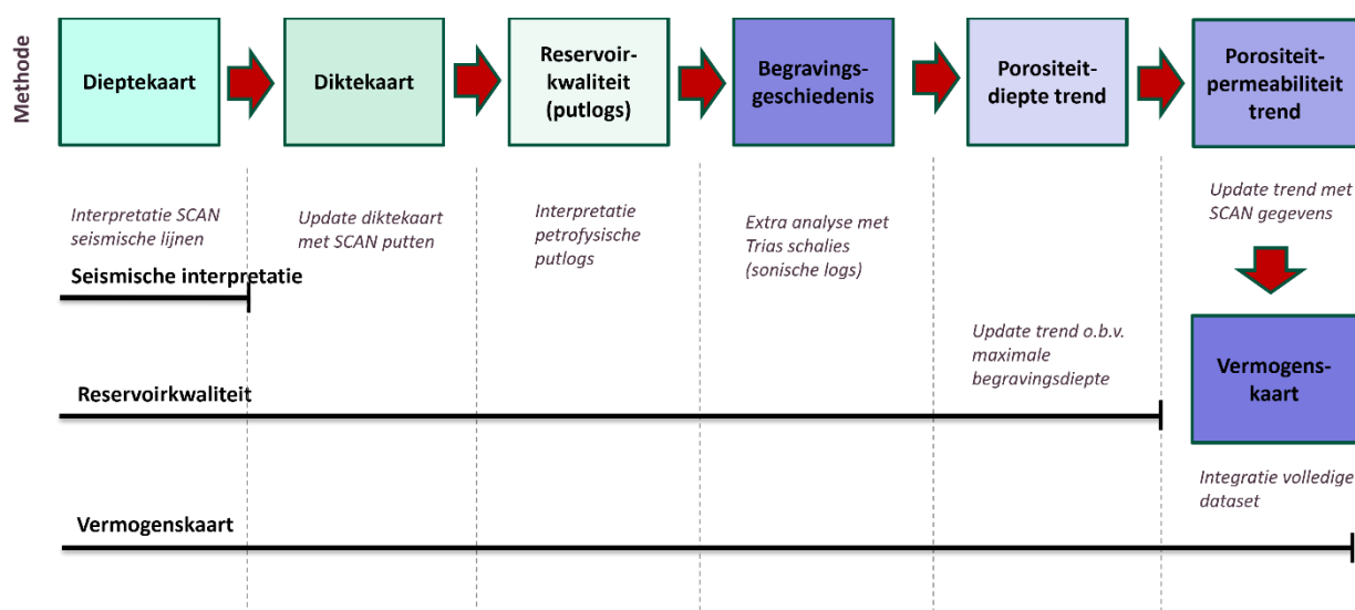
Figuur 5-1: Stappen gezet in dit onderzoek om tot een geothermische vermogenskaart te komen. Daarbij wordt gewerkt met data uit seismische interpretatie en putdata.
