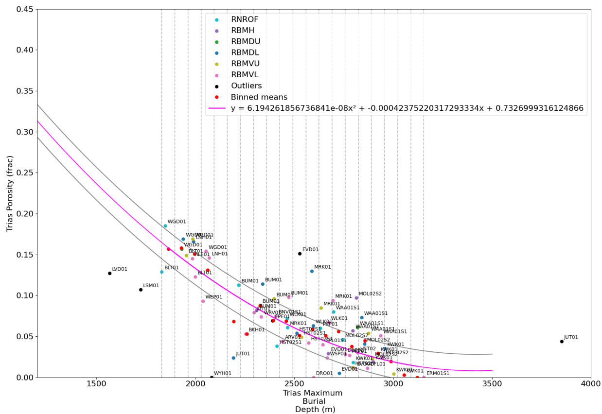
Figuur 3-17: Grafiek die de porositeit-diepte trend weergeeft voor de reservoirs van de Boven- en Onder Germaanse Trias Groepen-reservoirs (Trias), gebruikmakend van voor opheffing gecorrigeerde gemiddelde reservoirdieptes.
