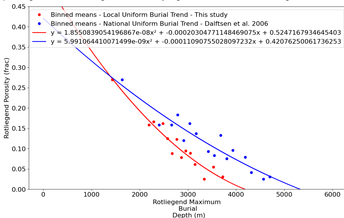
Figuur 3-19: Formatie van Slochteren (Rotliegend Groep) porositeit-diepte trends met behulp van de lokale begravingslijn gegenereerd in deze studie (rood) en de nationale (Dalftsen et al 2006) begravingslijn (blauw).
