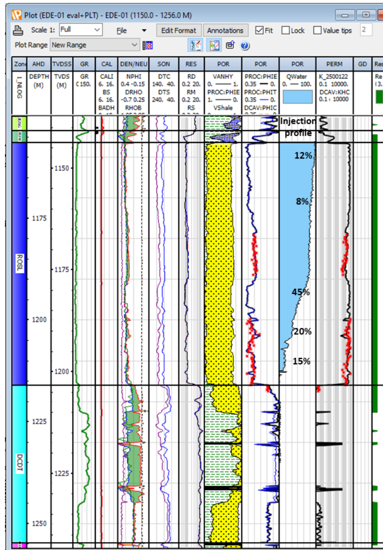
Figuur 3-22: Logplot van ROSL-interval in EDE-01 met open boorgatlogs track 4-8, geëvalueerde lithologietrack 9, porositeitstrack 10, PLT-injectieprofiel tijdens puttest track 11 en permeabiliteitstrack 12. Injectiepercentage per interval weergegeven in track 11.
