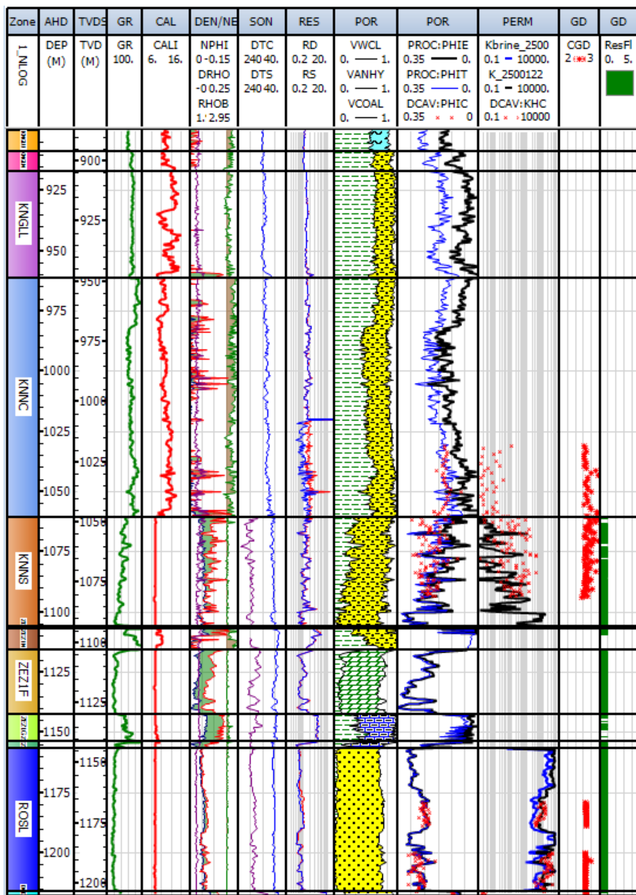
Figuur 3-26: Logplot met evaluatieresultaten voor SCAN-put EDE-01. Tracks 1-3 tonen zones, gemeten diepte en TVD's, tracks 4-7 bewerkte logs, track 8 lithologie, track 9 log/boorkernporositeit, track 10 log/ boorkernpermeabiliteit.
