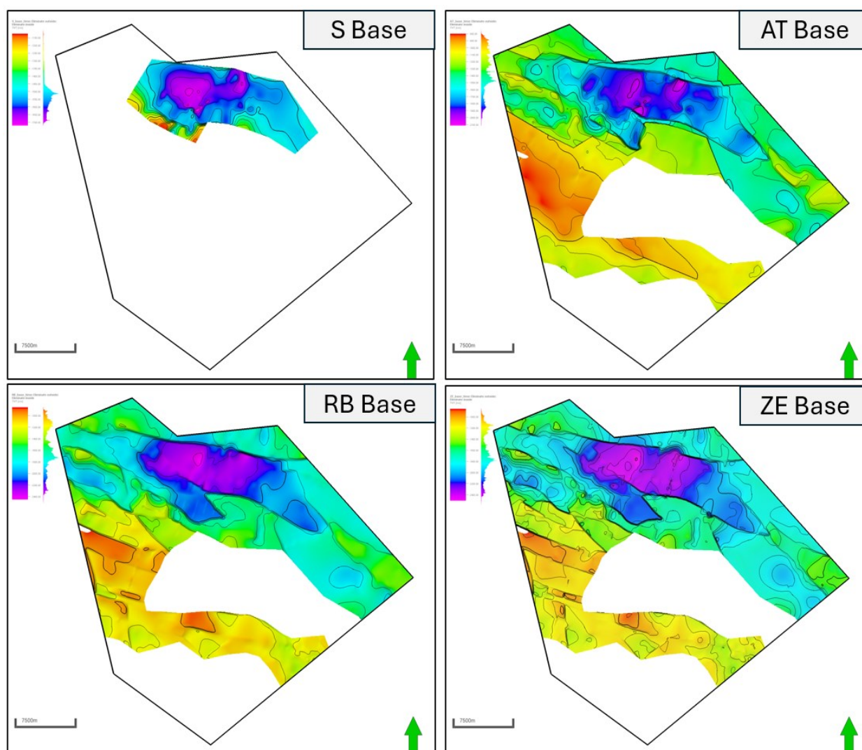
Figuur 2-3: Resulterende grids in het tijdsdomein (ms) voor Basis Schieland Groep (S), Basis Altena Groep (AT), Basis Onder-Germaanse Trias Groep (RB) en Basis Zechstein Groep (ZE).
