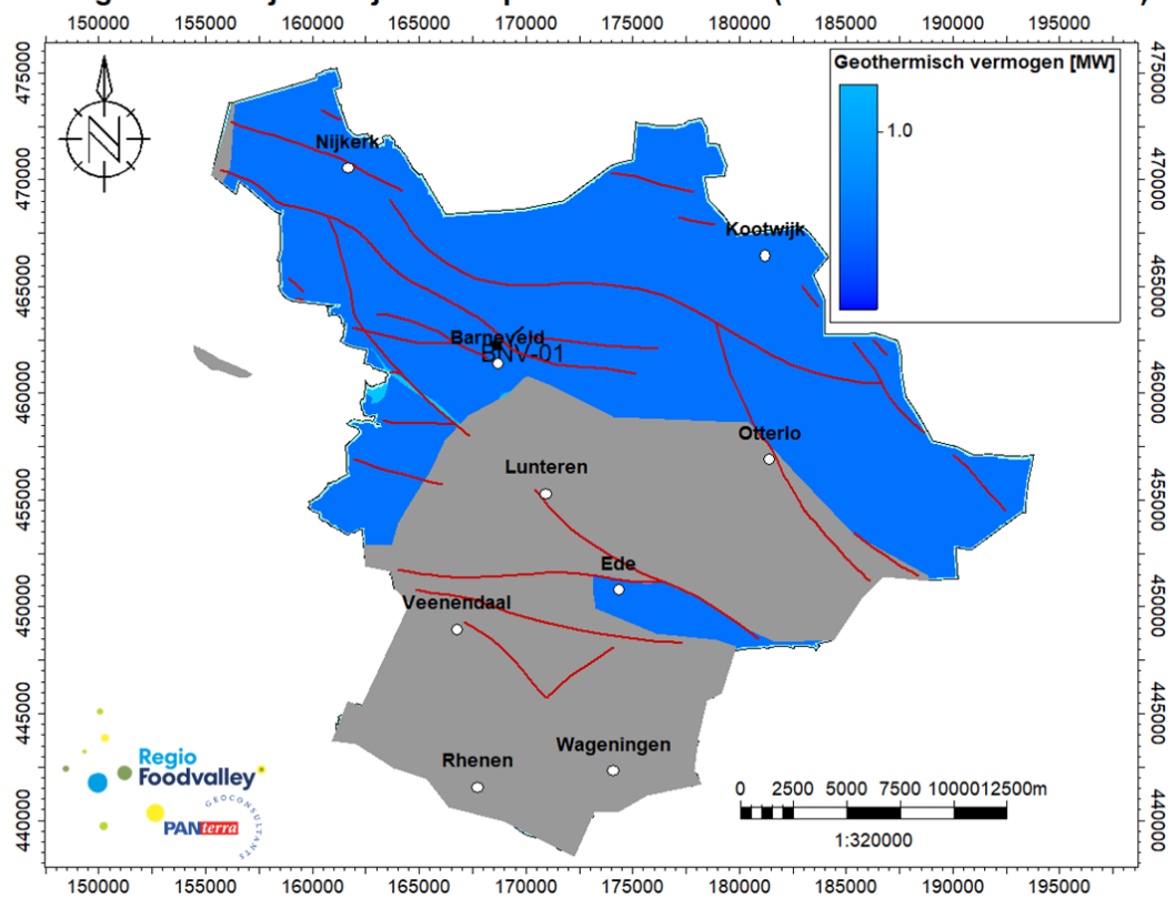
Vermogenskaart bij een injectietemperatuur van 15 °C (RBMVL - Middel scenario)
