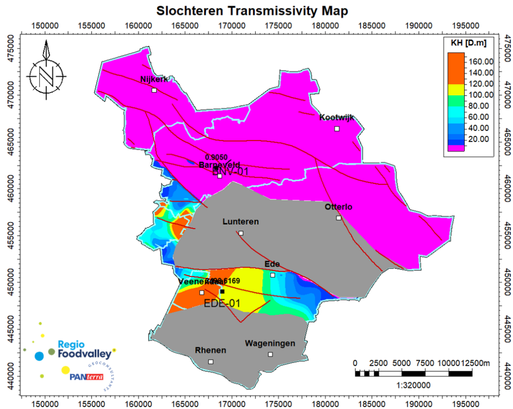
Figuur 5-4: Transmissiviteitskaart (= reservoirdikte * permeabiliteit) voor het Slochteren reservoir in het middel scenario. Rode lijnen geven breuken weer; grijze vlakken markeren gebieden waar de Formatie van Slochteren reservoir ontbreekt (op basis van seismische lijnen).
