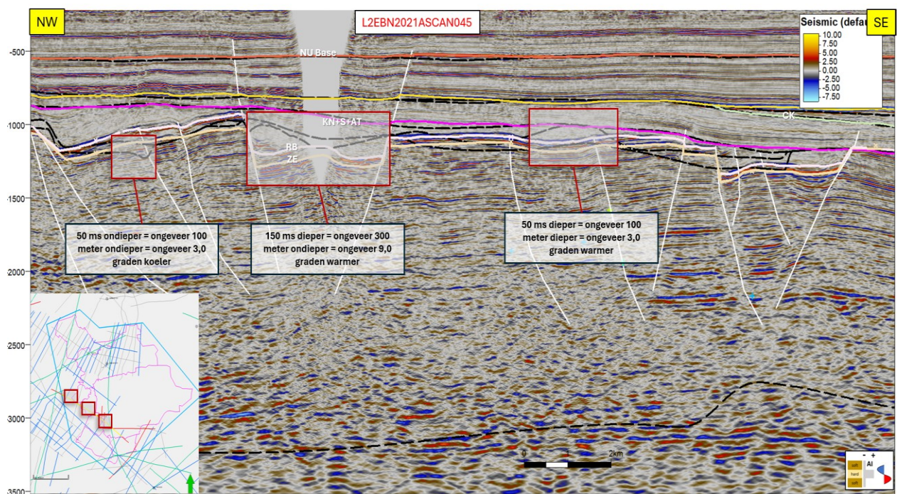
Figuur 2-14: Seismische lijn L2EBN2021ASCAN045 illustreert de vergelijking tussen oude (zwart) en bijgewerkte (gekleurd) interpretaties. Er zijn aanzienlijke verbeteringen rond breuken met verschillen van ongeveer 50-150 ms.
