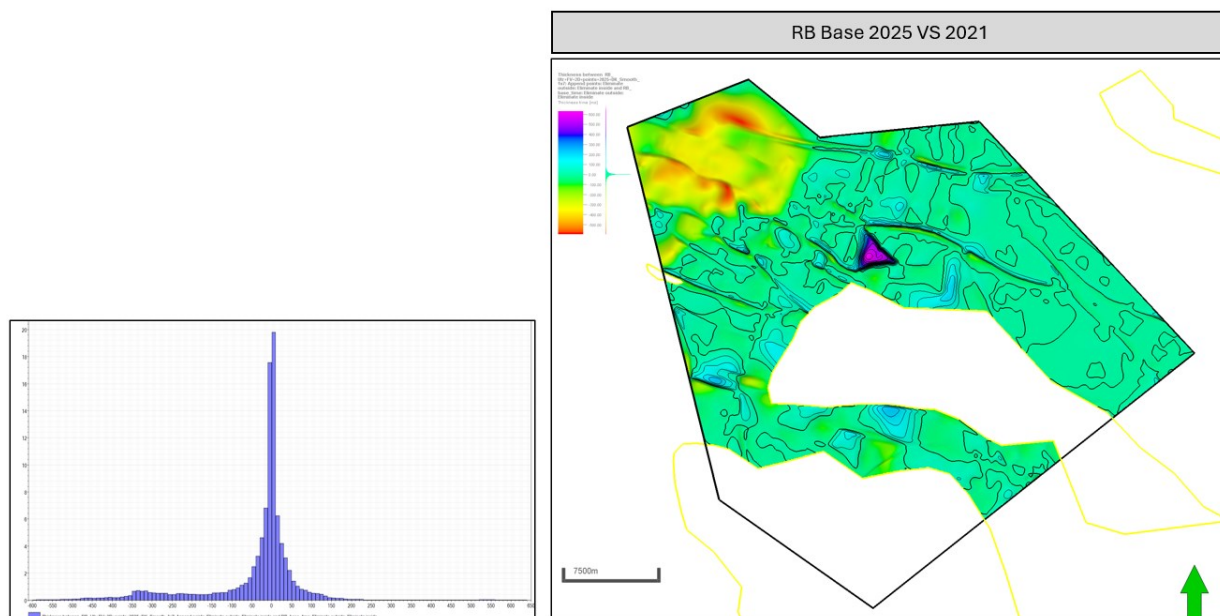
Figuur 2-12: Basis Onder-Germaanse Trias Groep (RB). Vergelijking tussen de seismische interpretatie van 2025 en het oude raster. Warme kleuren geven gebieden aan waar de bijgewerkte interpretatie dieper is, terwijl koude kleuren gebieden aangeven waar deze ondieper is. Het histogram aan de linkerkant illustreert de verdeling van diepteverschillen (ms) over het onderzoeksgebied.
