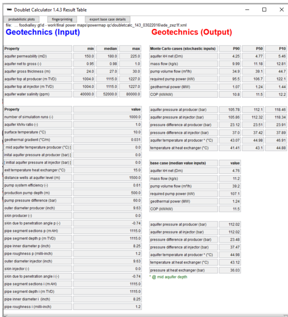
Figuur 4-9: DoubletCalc1D simulatie voor het ZE21F Randcarbonaat, op basis van de reservoir-eigenschappen bij EDE-01.
