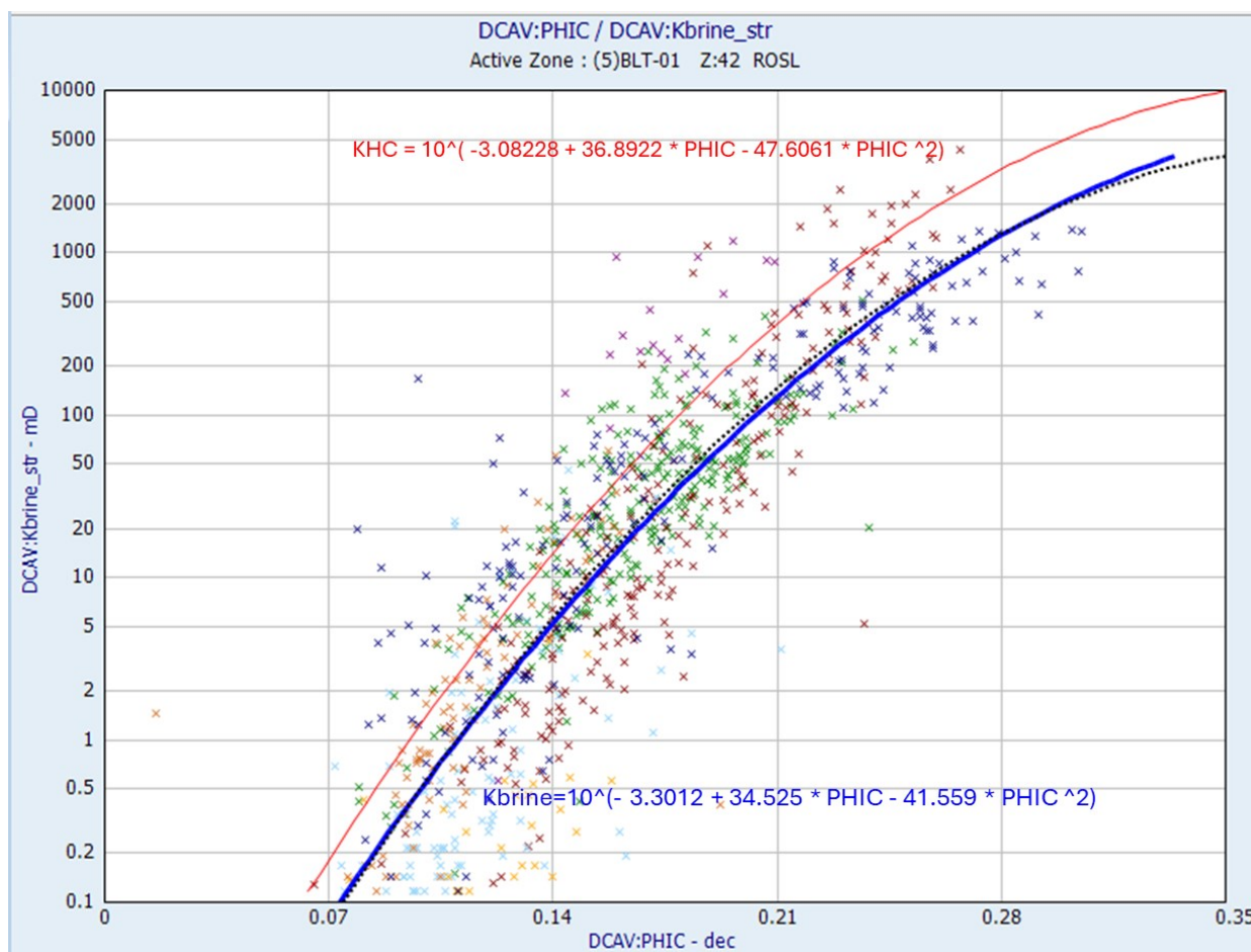
Figuur 3-14: Grafiek van de stressgecorrigeerde brijnpermeabiliteit, geschat op basis van SCAN-putcorrelatie, versus stressgecorrigeerde kernporositeit voor de ROSL. De weergegeven punten zijn per put gekleurd. Ook zijn de regressieaanpassing aan deze gegevens (blauwe curve) en de in-situ luchtpermeabilitetrend (rode lijn) weergegeven. De zwarte stippe lijn is de luchtpermeabilitetrend die is verschoven om overeen te komen met de brijntrend, ter illustratie van de schaalbaarheid.
