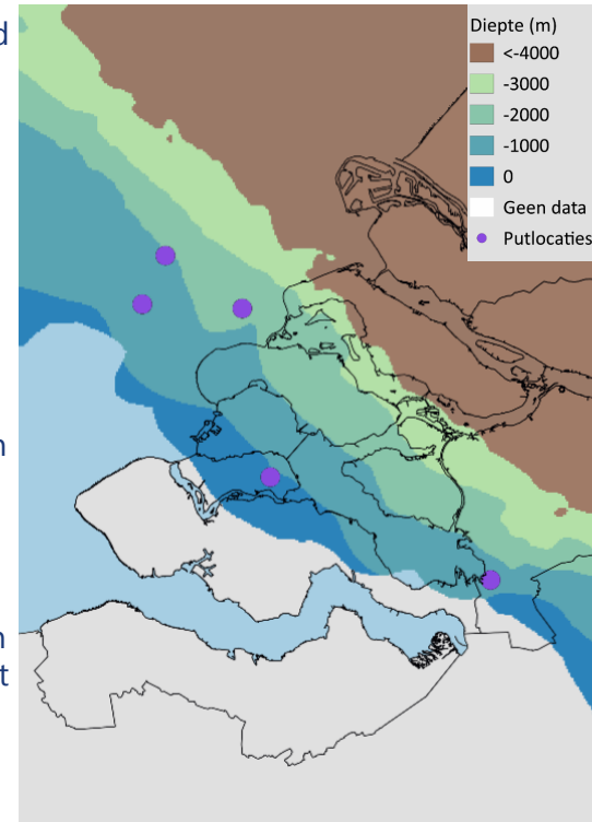
Kaart 11: Dieptekaart van het Dinantien.
