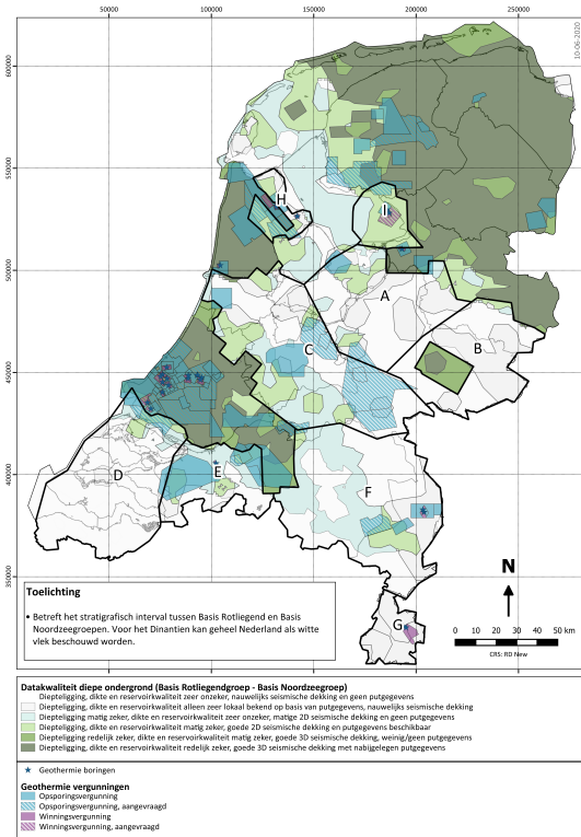
Kaart 14: SCAN-gebieden
