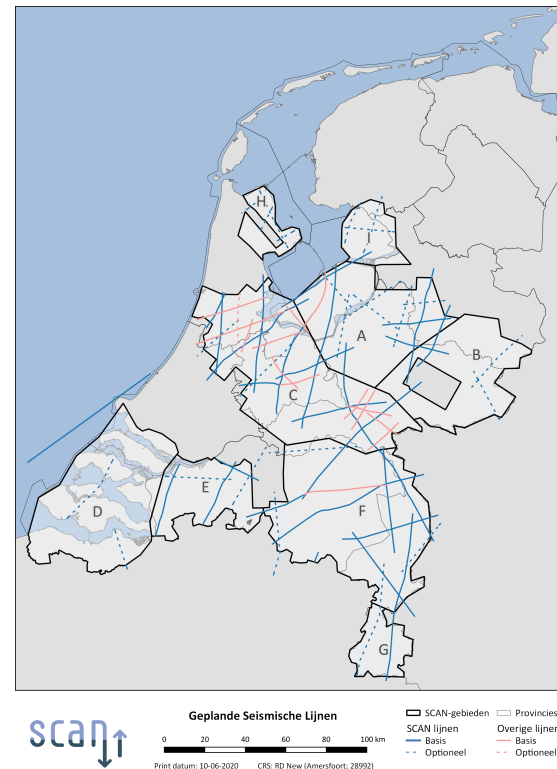
Kaart 15: SCAN-onderzoeksgebieden
