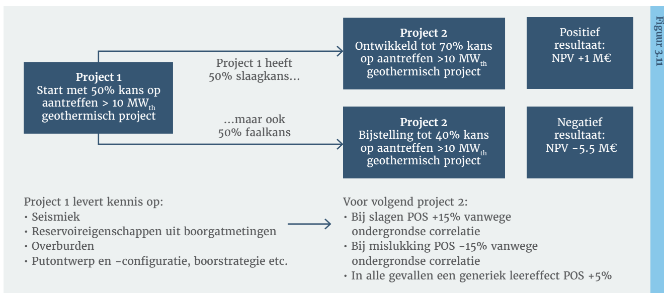
Figuur 3.11 Leer- of deriskeffect van project 1 voor vervolgproject 2 met een initiële startkans P50 vermogens-verwachtings waarde op het benodigde vermogen voor een gezond economisch project. Het slagen of falen van het eerste project heeft een belangrijke waarde-effect op de verwachting van het tweede en verdere projecten.
